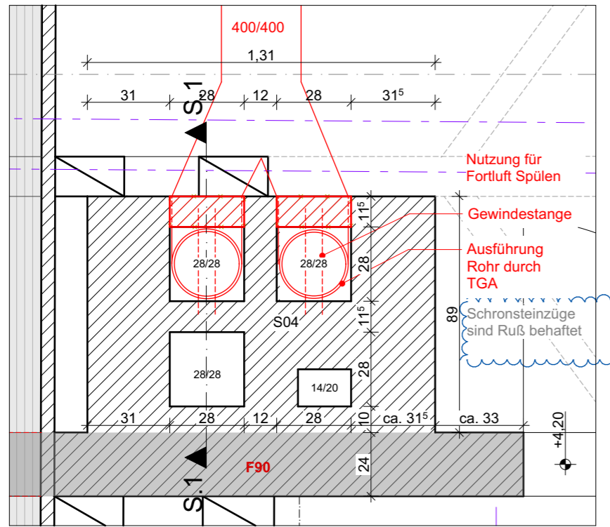
Grundriss Ausschnitt 1.OG M 1:20
