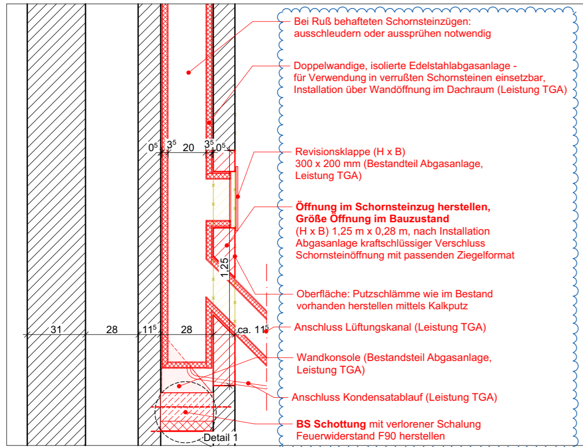
Schnitt 1 - S04 M 1:20
