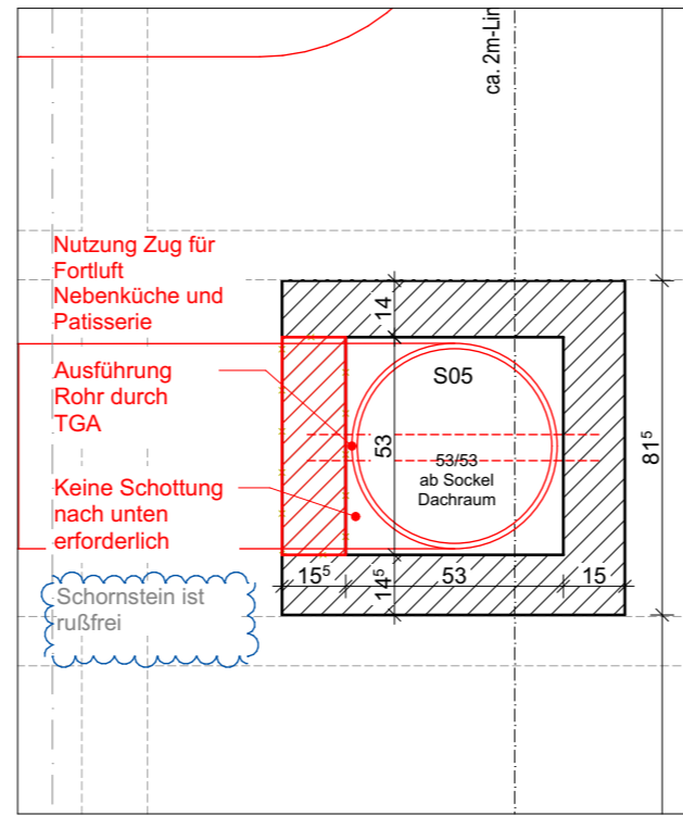
Grundriss Ausschnitt 1.OG M 1:20
